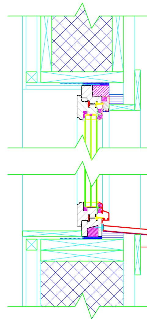
WOOD FRAME (VAPOR OPEN)
